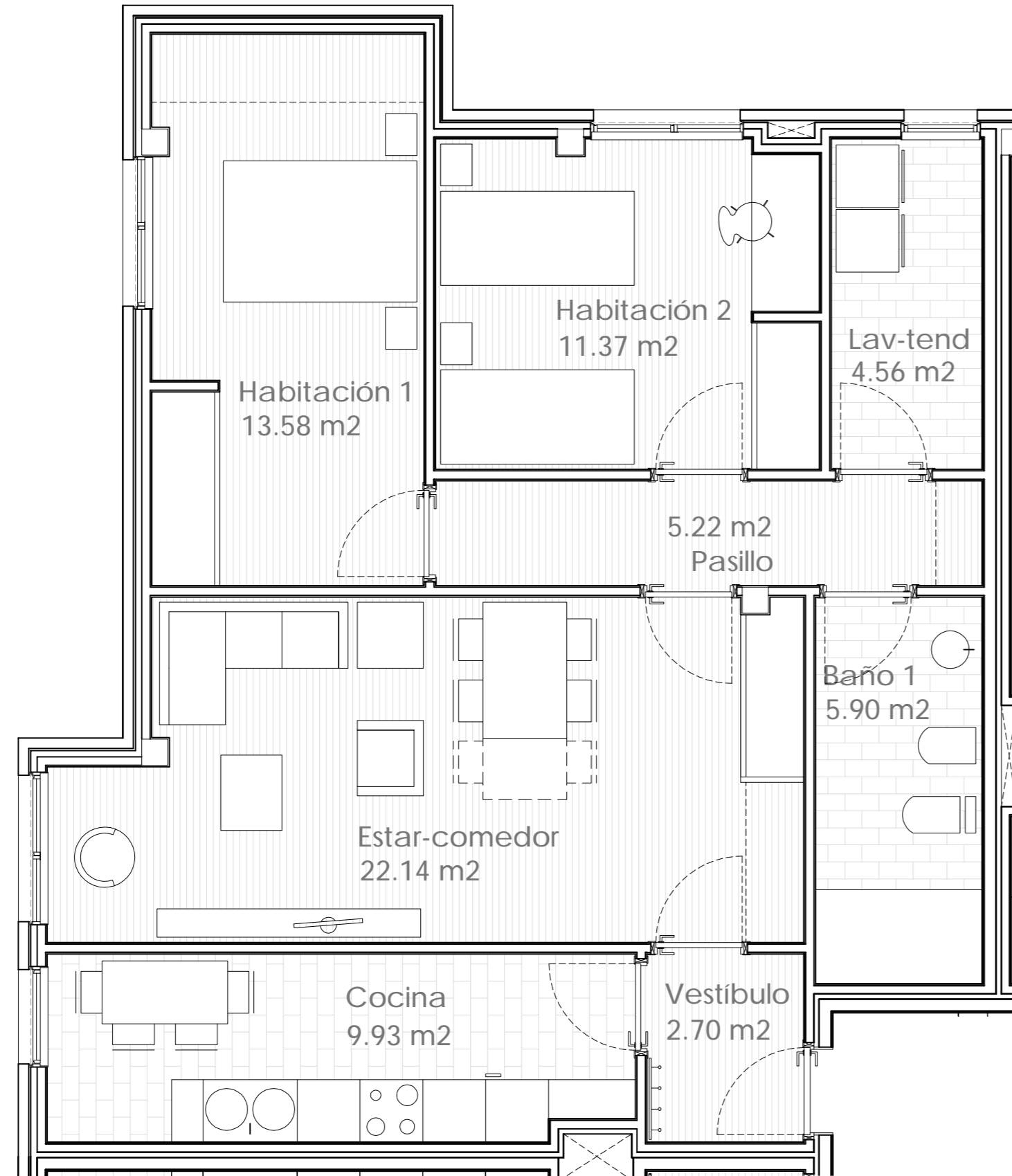
VIVIENDA B1-P1-VA y B1-P2-VA . escala: 1/50. Usos y superficies
