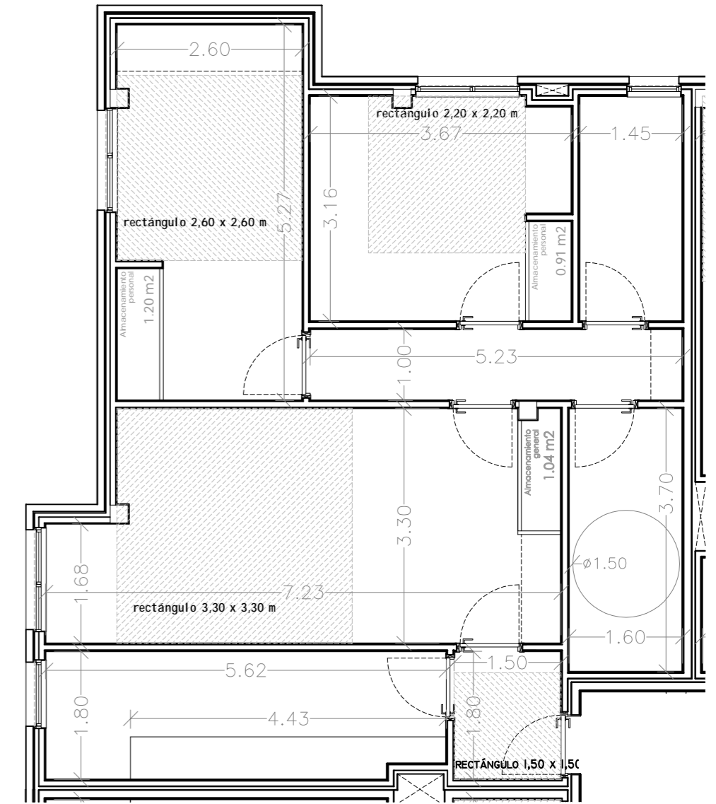
VIVIENDA B1-P1-VA y B1-P2-VA . escala: 1/75. NHV y cotas
