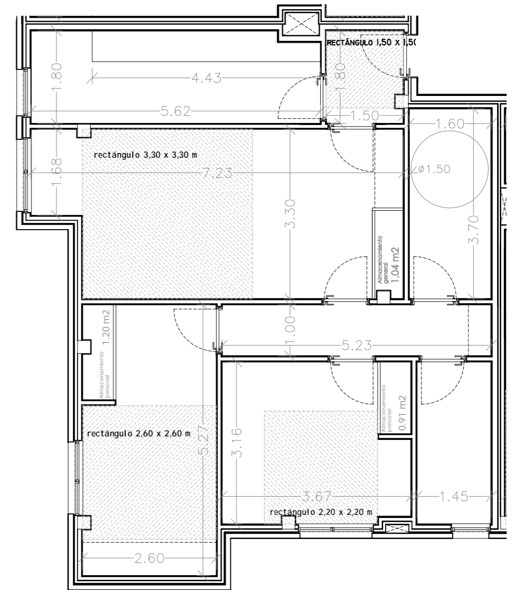
VIVIENDA B1-P1-VB y B1-P2-VB . escala: 1/75. NHV y cotas
